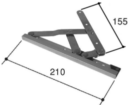
本図は右勝手 PKE5318R
