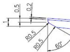
A部詳細 (5:1)
